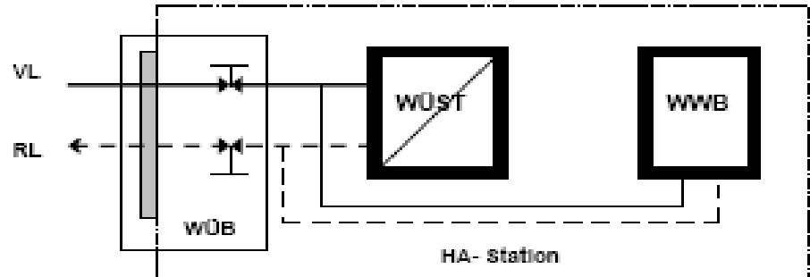
Abbildung 1: Schema Hausanschluss
